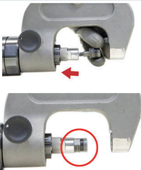
Matrize / Nietunterstützung
