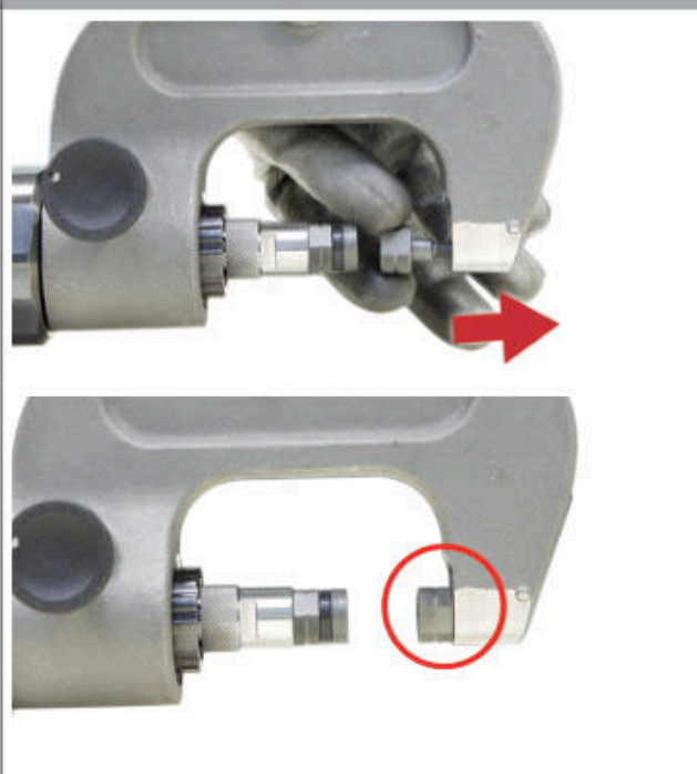
Матрица заклепки
